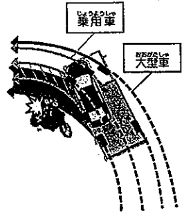
乗用車の内輪差：斜線部分 大型車の内輪差：色付き部分
